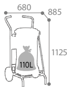
Roues pneumatiques
