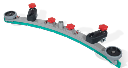
Suceur complet aluminium Roues réglables et lames en polyuréthane vert incluse TGB3045 / HGB3045 / TT4045G / TGB4045 / CRG8055 / CRG8072 / TTV678G (650) réf : 904691 TT4055G / TGB4055/T / TGB6055/T / TGB8572 (720) réf : 904699 - TTV678G (850) réf : 904694
